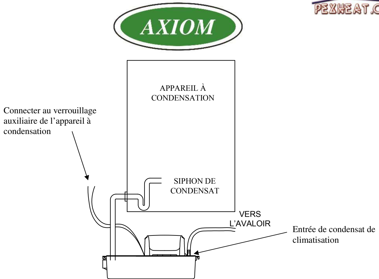
Figure 7 – Schéma d'installation du NT1-P
