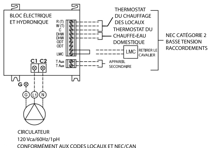
Figure 6 - Raccordement du thermostat et du circulateur
